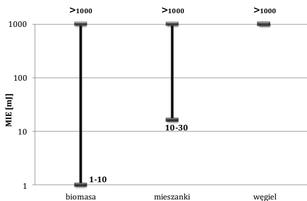
Rys. 7. Porównanie minimalnej energii zapłonu pyłu dla biomas, mieszanek biomas z węglami energetycznymi oraz węgla energetycznych
